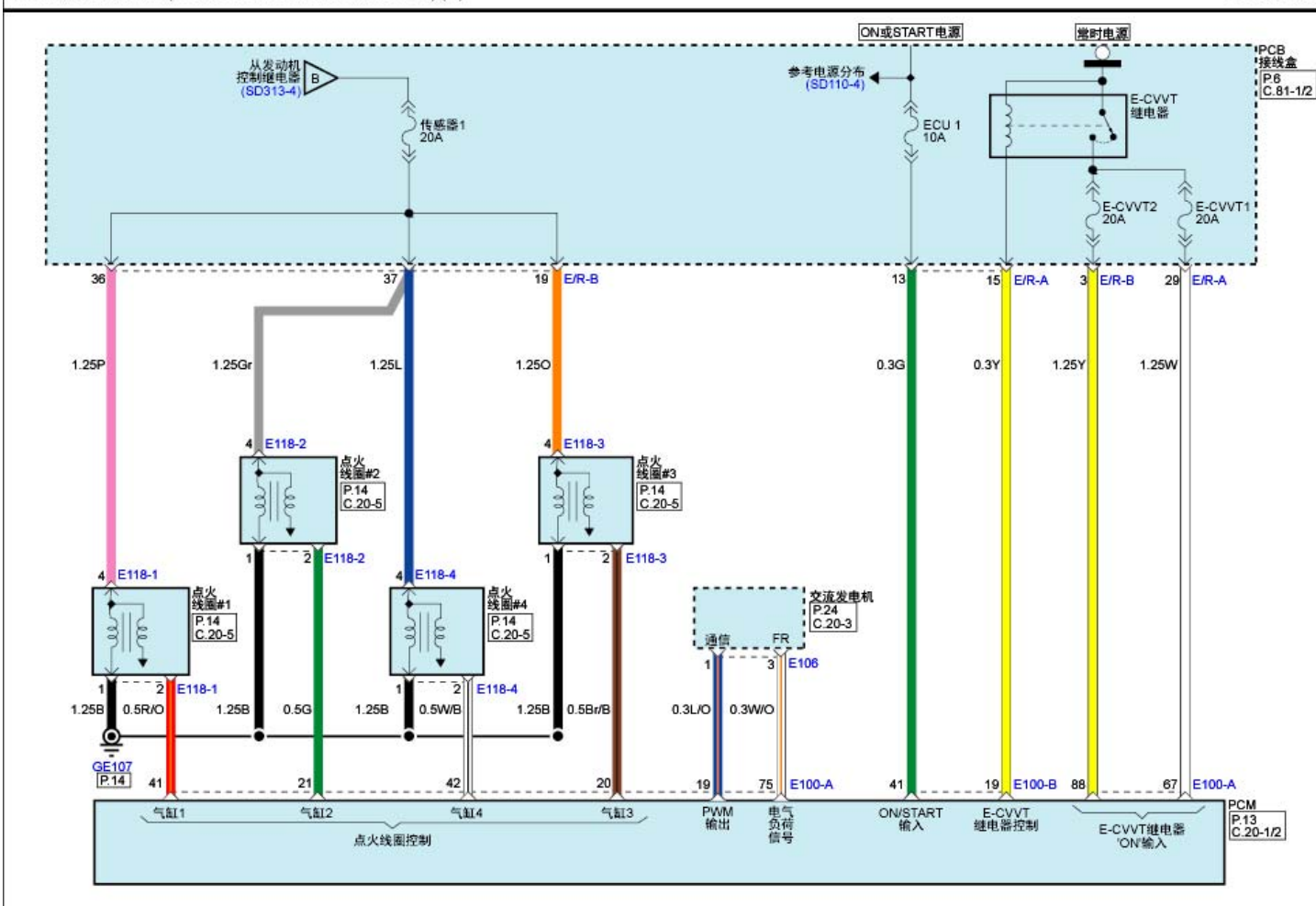
发动机控制系统(G4KJ: THETA-II 2.4L GDI)(5)
